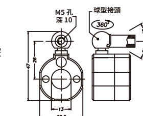
游標 (B) PCUR033
